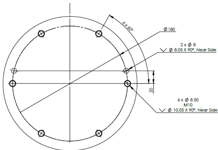
1.1: ロボットベースの底面図
