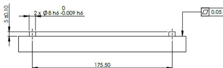
1.2: ロボットベース用取り付けプレート
